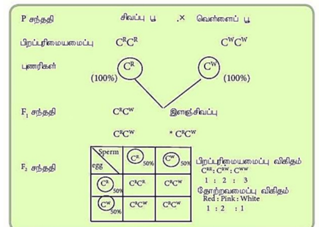
உரு 6.9. Mirabilis jalapa தாவர பூவின் நிறப் பரம்பரையலகில் நிறைவில் ஆட்சி
